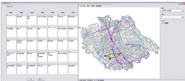
図 4: スケジューラ (左) とナビゲーション (右)
